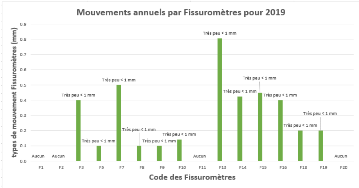
Histogramme 3 : Mouvements annuels par fissuromètre pour 2019
