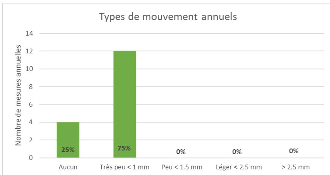
Histogramme 4 : Types des mouvements annuels des fissuromètre
